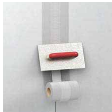
Aufbringen des fermacell Armierungsbandes HD
