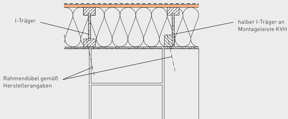
Horizontalschnitt
