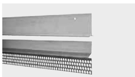
fermacell Deckenstoßprofil HD (mit Profiloberteil und -unterteil)
