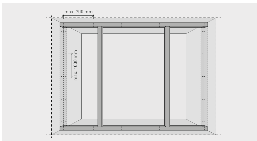
Befestigungsabstände
