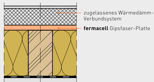
Wirksamer Wetterschutz WDVS
