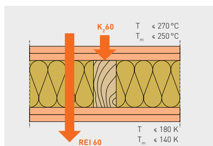
Beispiel Gebäudeklasse 4: Ausführung einer Holzständerwand (REI 60/K 2 60) gemäß den Anforderungen der Muster-Richtlinie (M-HFHolzR)/hochfeuerhemmendes Bauteil
