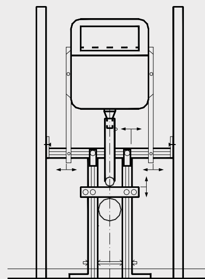
Tragständer für wandhängende WCs mit Einbauspülkästen
