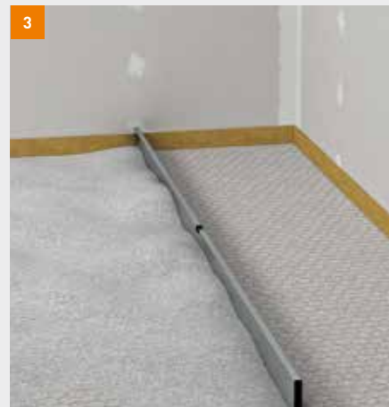
fermacell Wabenschüttung abziehen
