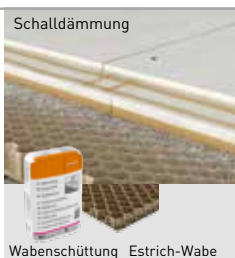
Wabenschüttung Estrich-Wabe
