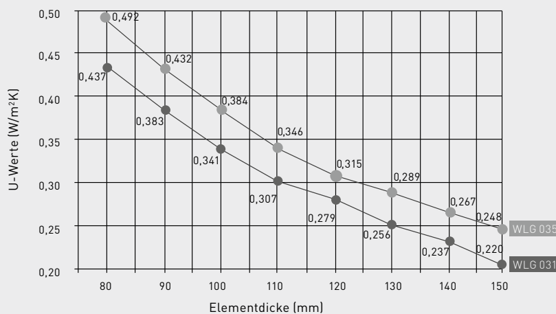
U-Werte der fermacell Dachboden-Dämmelemente N+F WLG 031 bzw. WLG 035 zur Berechnung beliebiger Rohdecken
