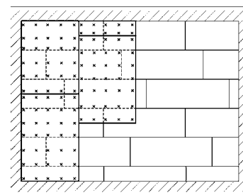
Verlegeschema 3. Lage
