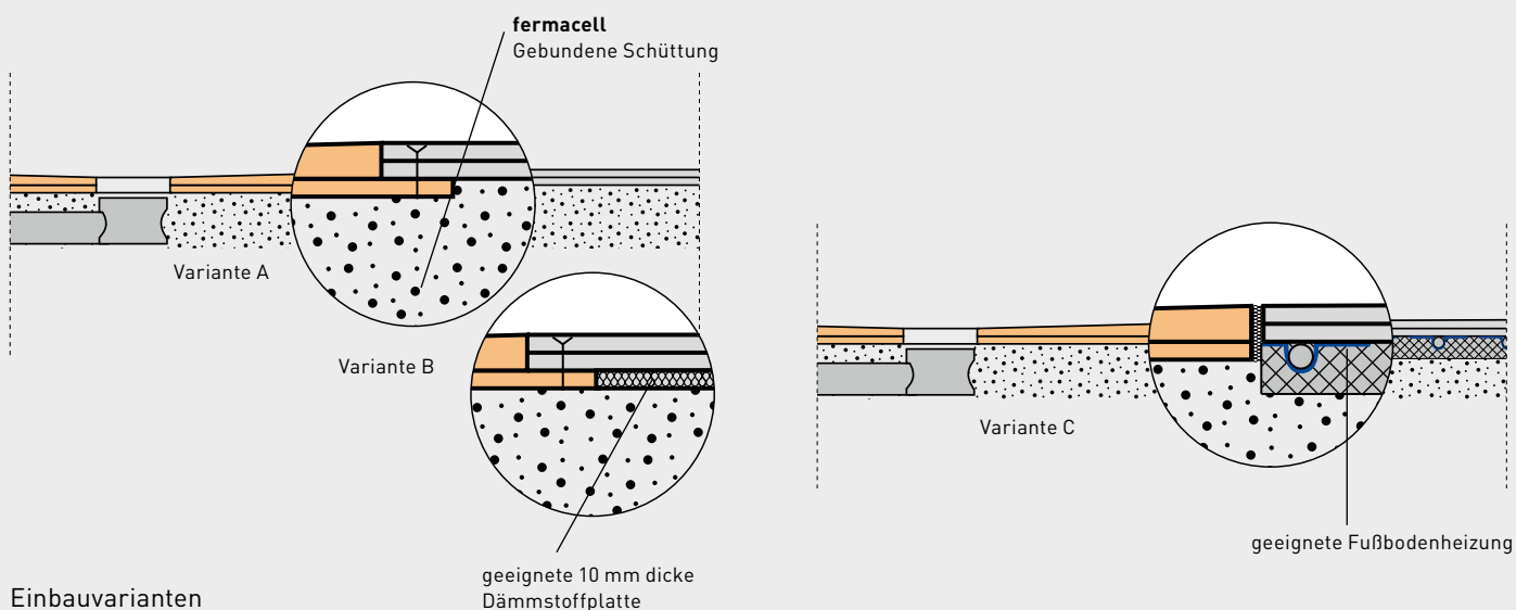
Beispiel: Wand – Fußbodenanschluss
