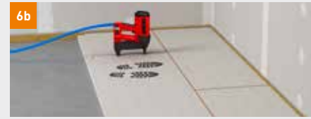
6a 6b Befestigen durch Verschrauben oder Spezial-Spreizklammern innerhalb von 10 Min.
