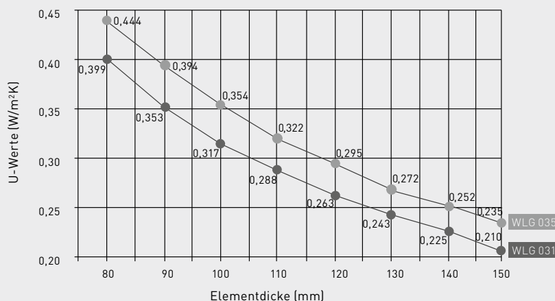
U-Werte [W/m 2 K] der mit fermacell Dachboden-Dämmelementen N+F WLG 031 bzw. 035 gedämmten Betondecke
