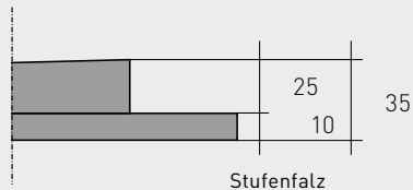
Beispiel Duschelement 1000×1000 mm
