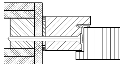
Montagewand
