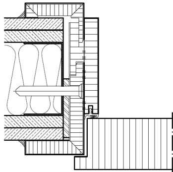
Montagewand
