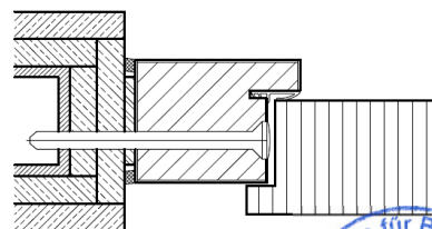
bekl. Stahlstütze
