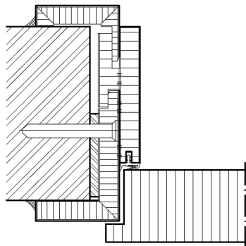
Holzstütze
