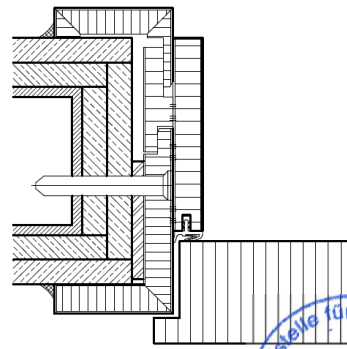
bekl. Stahlstütze
