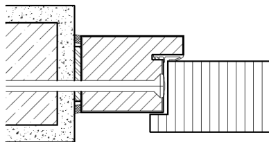
Massivwand
