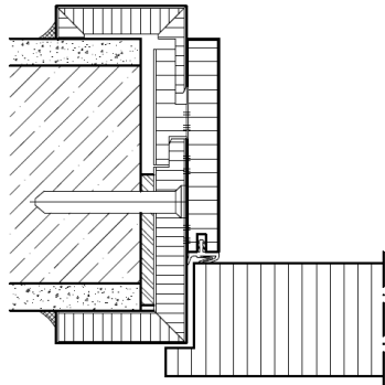
Massivwand
