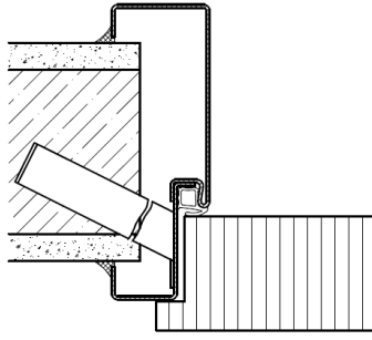
Massivwand
