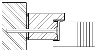
Holzstütze
