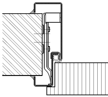
Holzstütze
